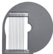
TAG02020 Mod. B6 6 mm N. LIST 2 da abbinare al disco E6 combine with E6
