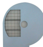
TAG03021 Mod. D 12x12 12 mm N. LIST 263 da abbinare al disco E14 combine with E14
